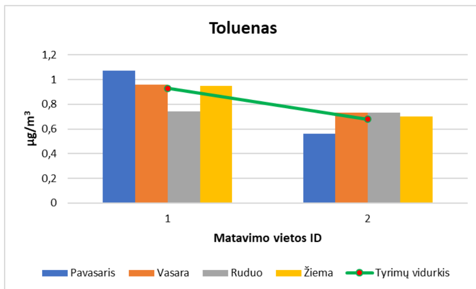
9 pav. Tolueno koncentracijų pasiskirstymas Šakių rajone, nustatytose matavimų vietose. (Ribinė vertė 600 \mu\text{g}/\text{m}^3 grafike neatvaizduojama, nes gautos tolueno koncentracijos ženkliai mažesnės už ribinę vertę)
