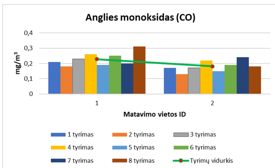
14 pav. CO koncentracijų pasiskirstymas Šakių rajone, nustatytose matavimų vietose. (Ribinė vertė 10 \text{mg}/\text{m}^3 grafike neatvaizduojama, nes gautos CO koncentracijų vertės ženkliai mažesnės už ribinę vertę)
