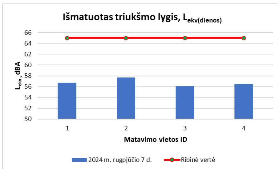
26 pav. Ekvivalentinio triukšmo pasiskirstymas matavimų vietose dienos metu (7 – 19 val.).
