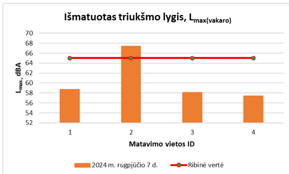
27 pav. Maksimalaus triukšmo pasiskirstymas matavimų vietose vakaro metu (19 – 22 val.).
