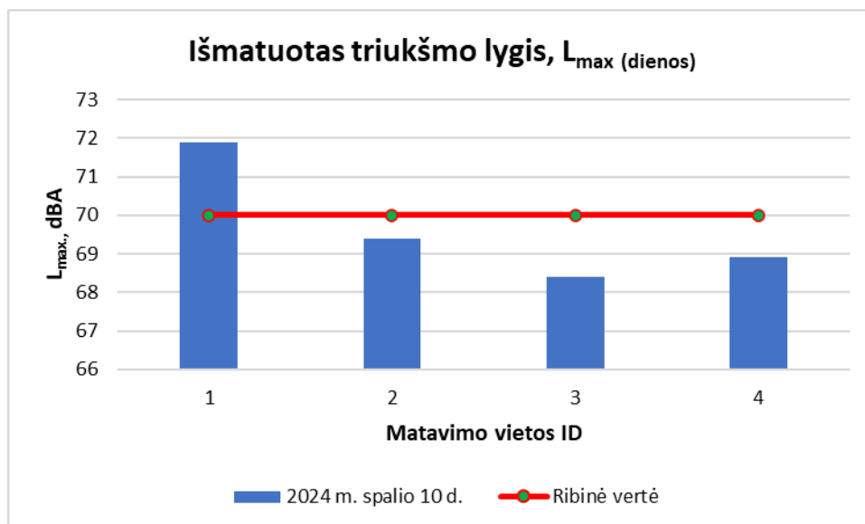
33 pav. Maksimalaus triukšmo pasiskirstymas matavimų vietose dienos metu (7 – 19 val.). Ribinis dydis 70 dBA
